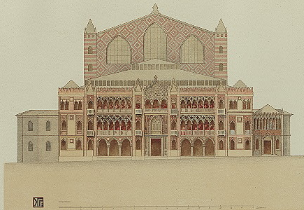
Проектъ театра для Тифлиса Державинъ и Покровскій Главный фасадъ
